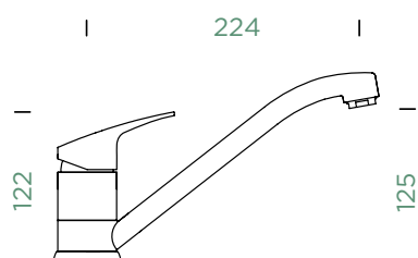
FESTAUSLAUF
