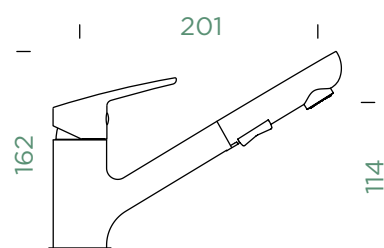
AUSZIEHBAR
